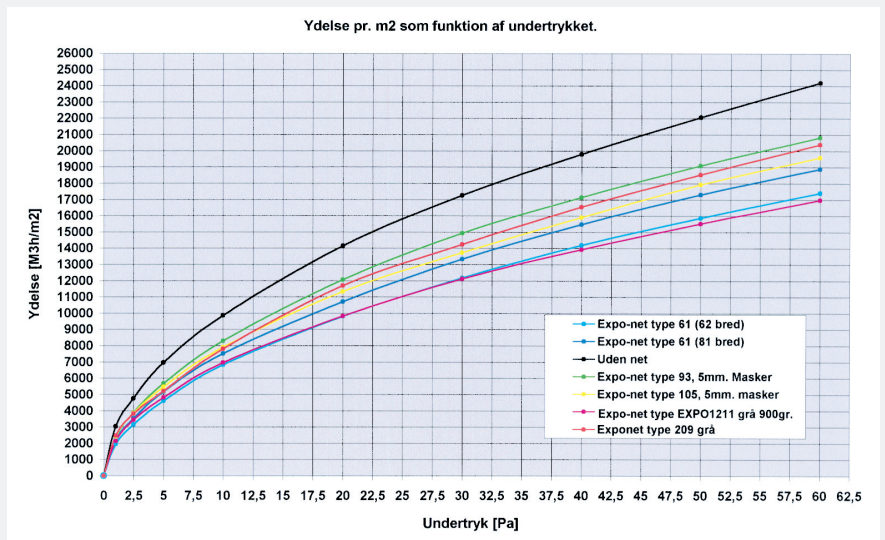
Tekniske målinger af vindbrydning udført på forskellige typer net.
