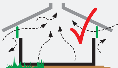
Eksempel på opbygning af moderne stalde, hvor nettet er monteret fra ydervæg til tag.
