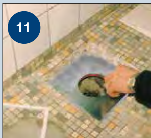
11 Tætningsmassen trækkes ind over flangen for at sikre forbindelse beton/flange.
