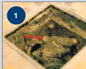
Eksempel på en tiltrængt renovering og hvor en nærmere undersøgelse viser, at der er huller i opstøbningen.
