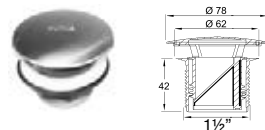
VVS nr. 747263-010
