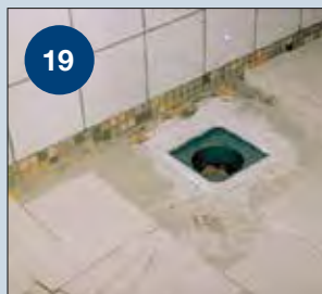
19 Afretningslag og fliseklæb kan nu påføres.
