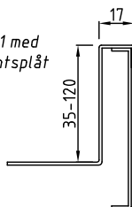
Droppkant 20 kakel
