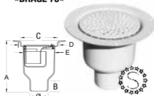
»BRAGE 75«
