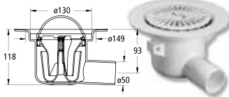
Mini Oden 50
