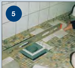
Renoveringssæt tilpasses færdig gulvhøjde.
