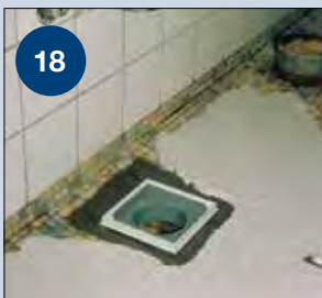
18 Afvent nu betonens færdige afhærdning før afretningslaget påføres.
