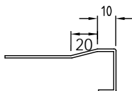
Droppkant 20 kakel
