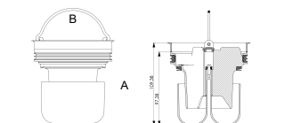
FlexNEPTUN®uden adapter-ring. Passer til ovenstående afløbsskåle
