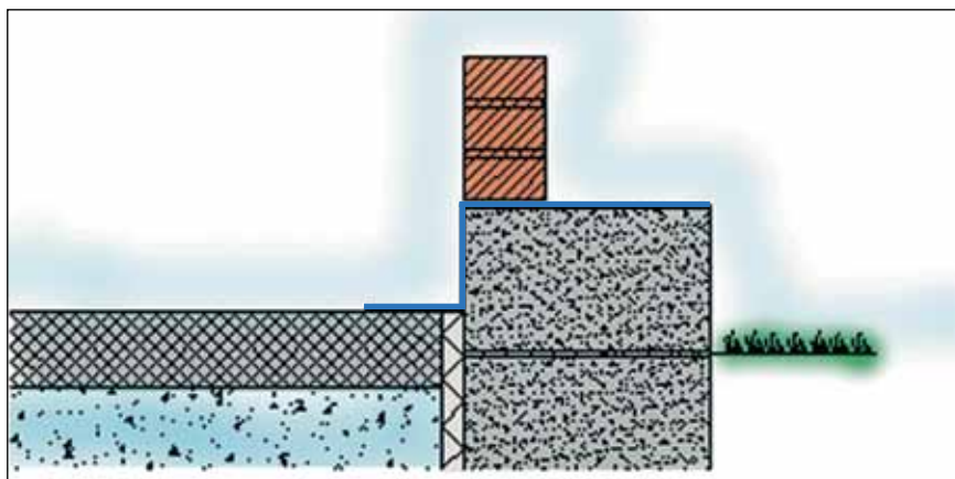
Vandafledende lag
