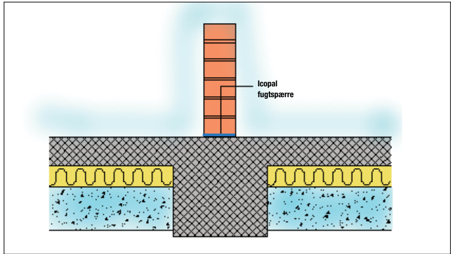
Skillevægge
