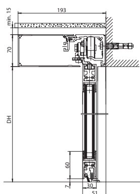
Lodret snit
