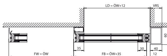
Vandret snit med 1 dørføj
