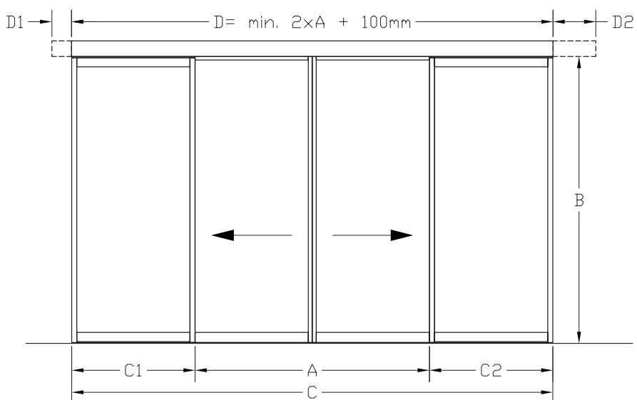
Opstalt – 2 fløjet med sideparti
