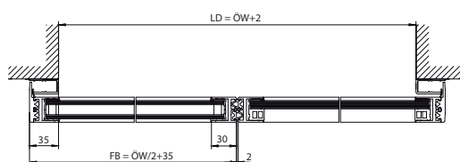
Vandret snit med 2 dørføj
