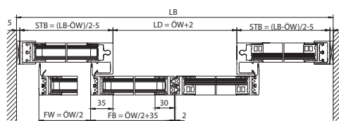
Vandret snit med sideparti
