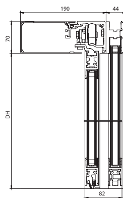
Lodret snit med bæreprøfil og sideparti
