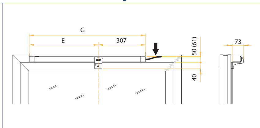
Pladskrav til INDADGÅENDE rammemontering
