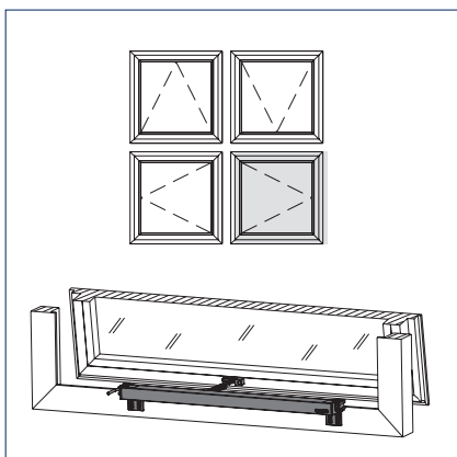
UDADGÅENDE rammemontering
