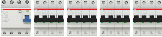
G4-3 HPFI-A 40A30mA + 1x4P 16A-C + 3x4P 13A-C
