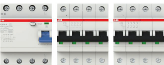
A1-2 HPFI-A 40A30mA + 2x4P 10A-C
