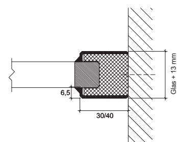
Vægttilslutning
