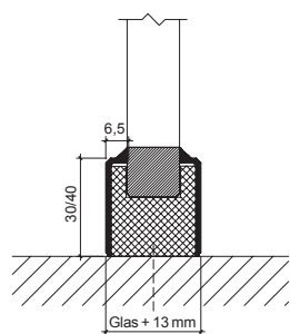
Gulvtilslutning
