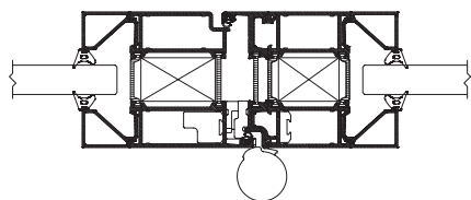
Glasrammedør aluminium
