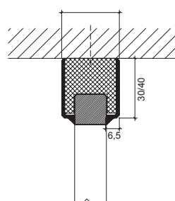
Lofttilslutning
