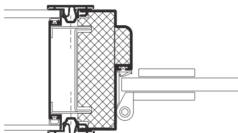
Helglasdør i DEKO GV glasvæg aluminiumindfatning type ASPD
