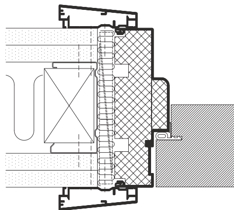
Lyddør i gipsvæg aluminiumindfatning type ASIF
