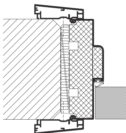
Dør i betonavæg aluminiumindfatning type ASIF
