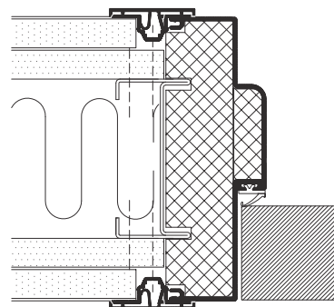
Dør i DEKO PF gipsvæg aluminiumindfatning type ASPD
