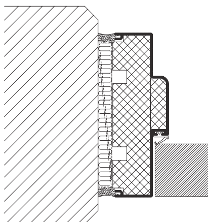
Dør i betonavæg - fugesamling
