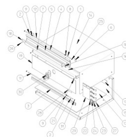
Løsdeler oversigt
