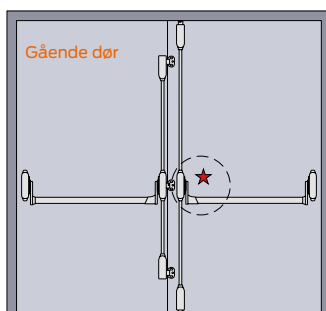
5-punktslukning - overfalsede
