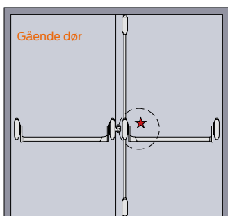
3-punktslukning - overfalsede
